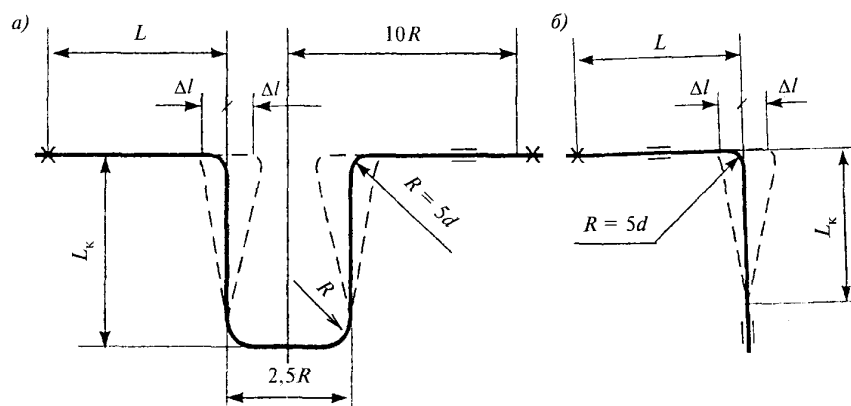
Рисунок 1 - Устройство П-образного (а) и Г-образного (б) компенсаторов
